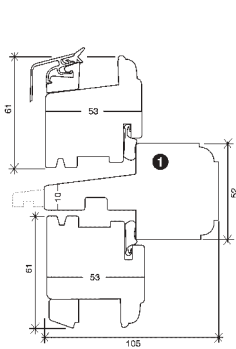
Tværpost m. alu bundglasliste
